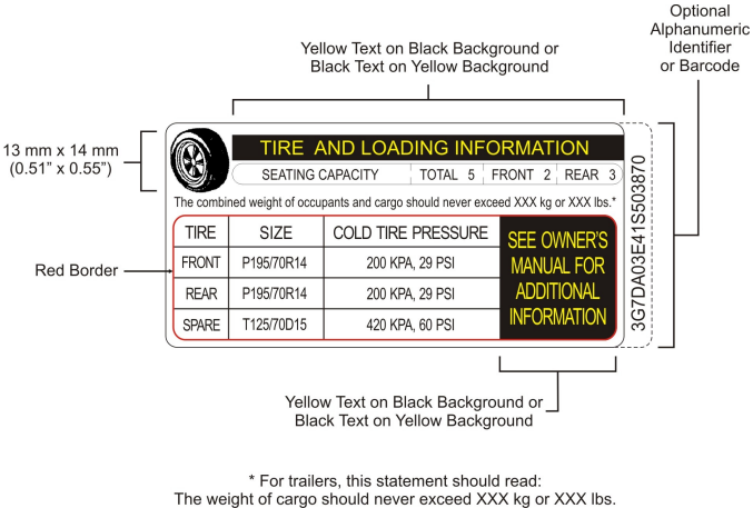
Figure 2 — exemple unilingue anglais de plaque de véhicule
