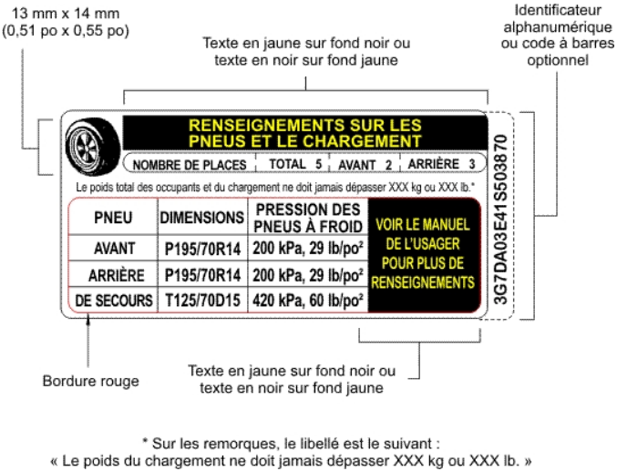
Figure 1 — exemple unilingue français de plaque de véhicule
