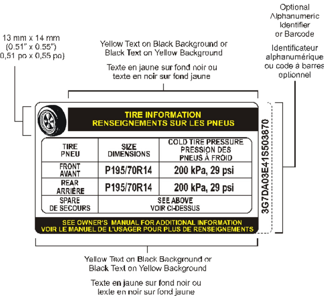
Figure 6 — exemple bilingue d'étiquette de pression de gonflage des pneus
