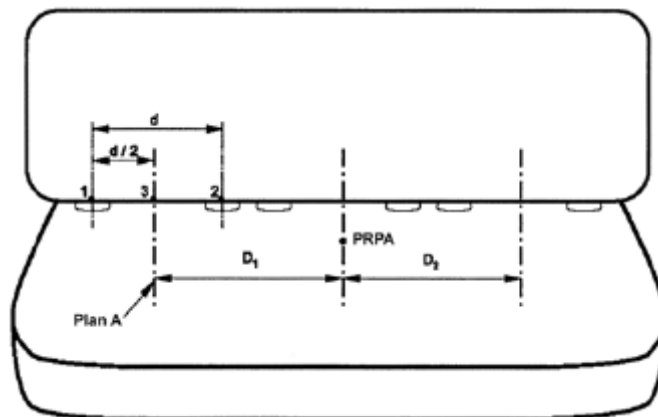
Figure 20 — Mesure de la distance entre les places assises désignées adjacentes à utiliser pour la mise à l'essai simultanée
