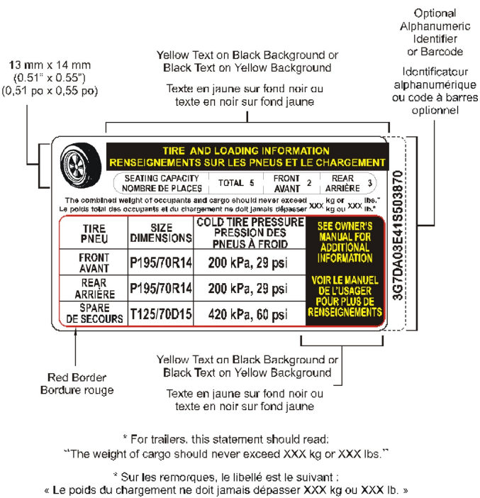
Figure 3 — exemple bilingue de plaque de véhicule
